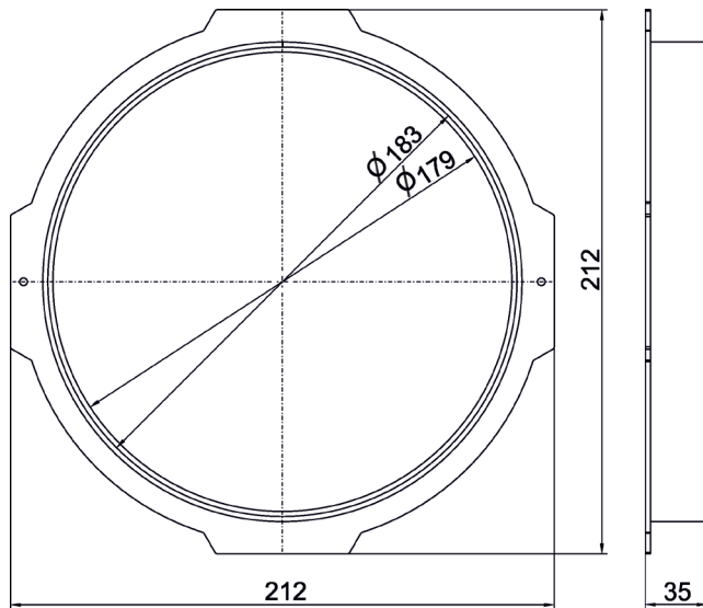
Top Hat 35 Esprite (P/N 10980568)
